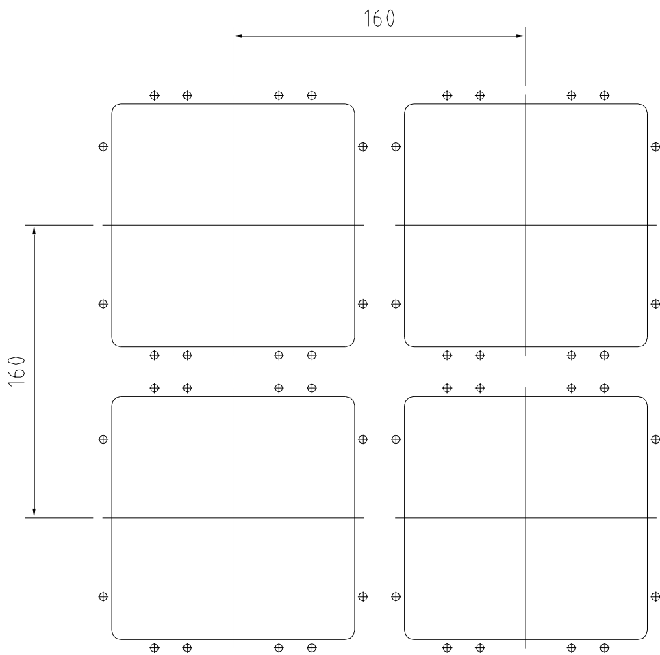
2By2 Array
